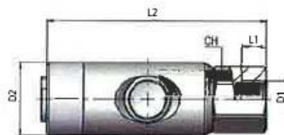
Innengewinde
